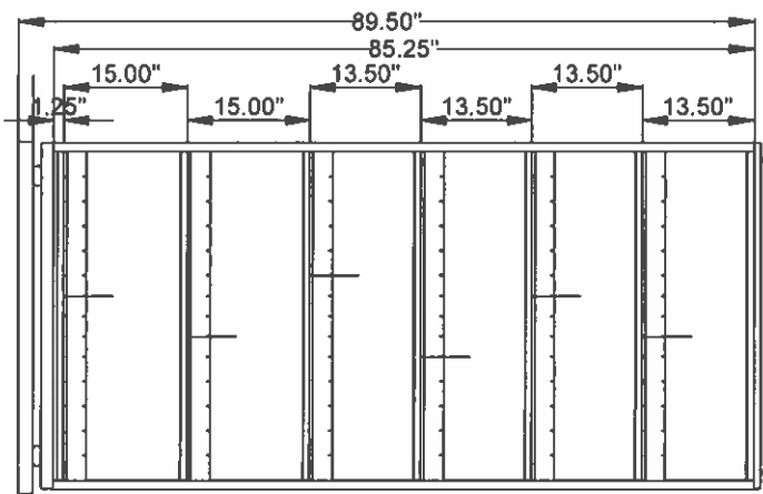
Elevation B
